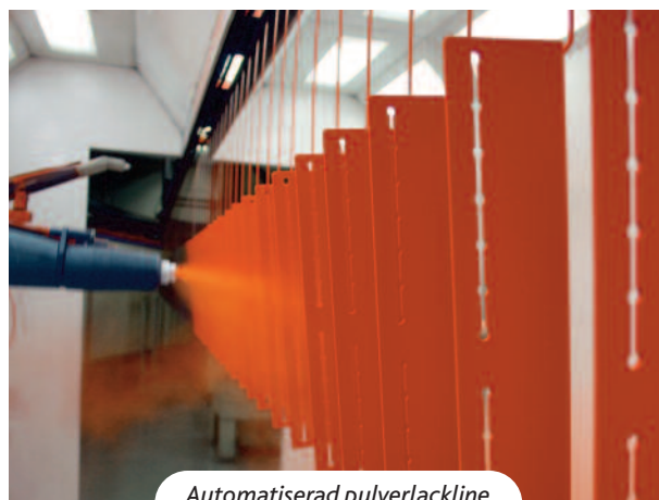
Automatiserad pulverlackline
